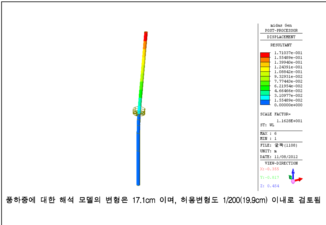
[해석 모델 변형도]
