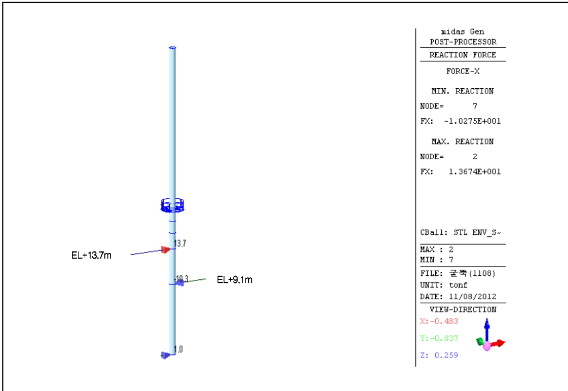
[해석모델 지점 반력도(X방향)]
